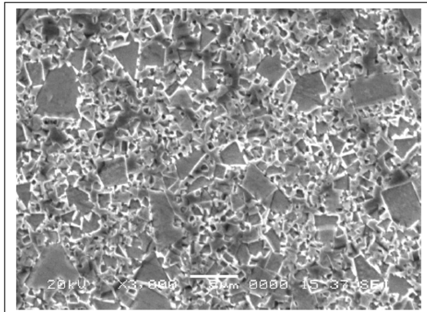
Microstruttura
